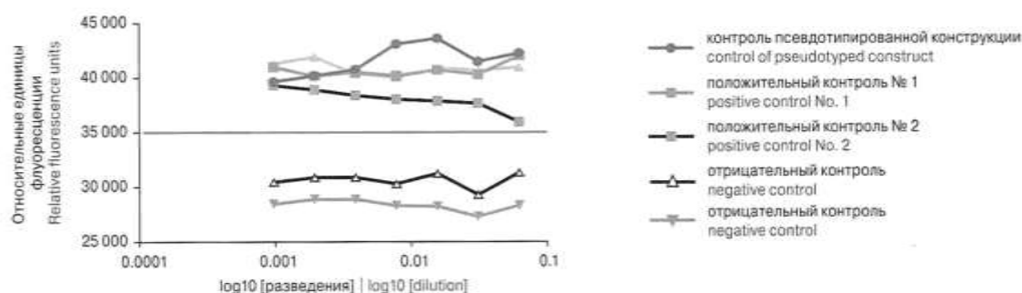
Рисунок 1. Детекция флуоресценции
